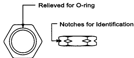
AN6289 B/H Nut
